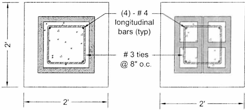
16"X8"X16" CMU (2) - 8"X8"X16" CMU Column Section Options
